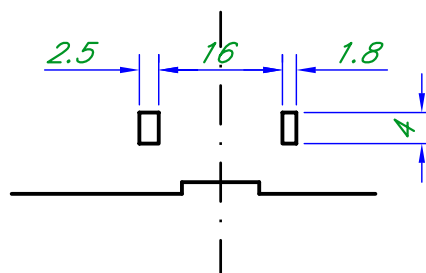
Foratura nominale
