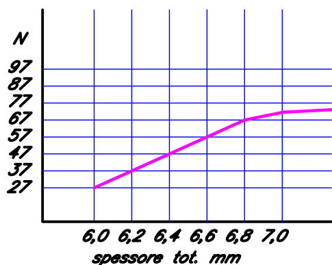
Curva caratteristica della molla
