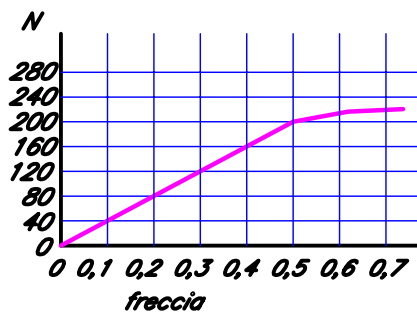
Curva caratteristica della molla
